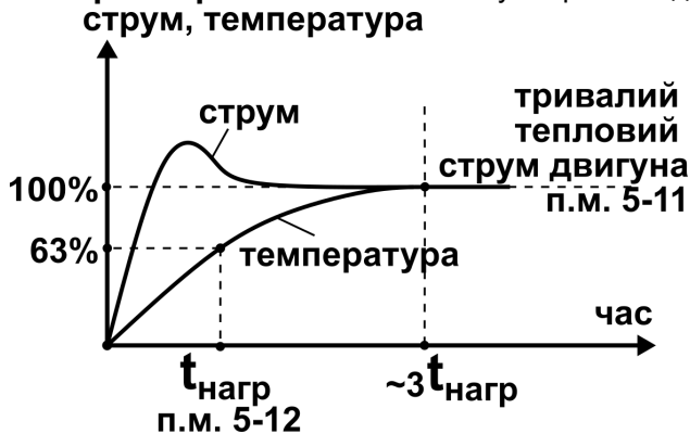
Рисунок 24. Вид перехідного процесу нагрівання електродвигуна.
