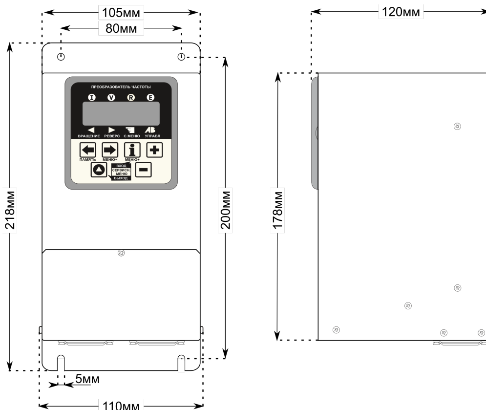
Рисунок 1а. Габаритні розміри перетворювачів CFM210 1.1 та 1.5кВт.
